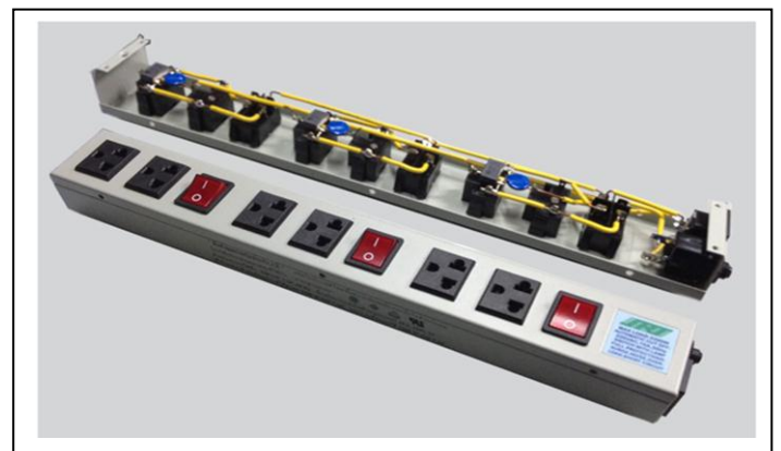
No. PC-63U 3สวิตช์คุ่ม 3 จุด เต้ารับ 6 ที่
